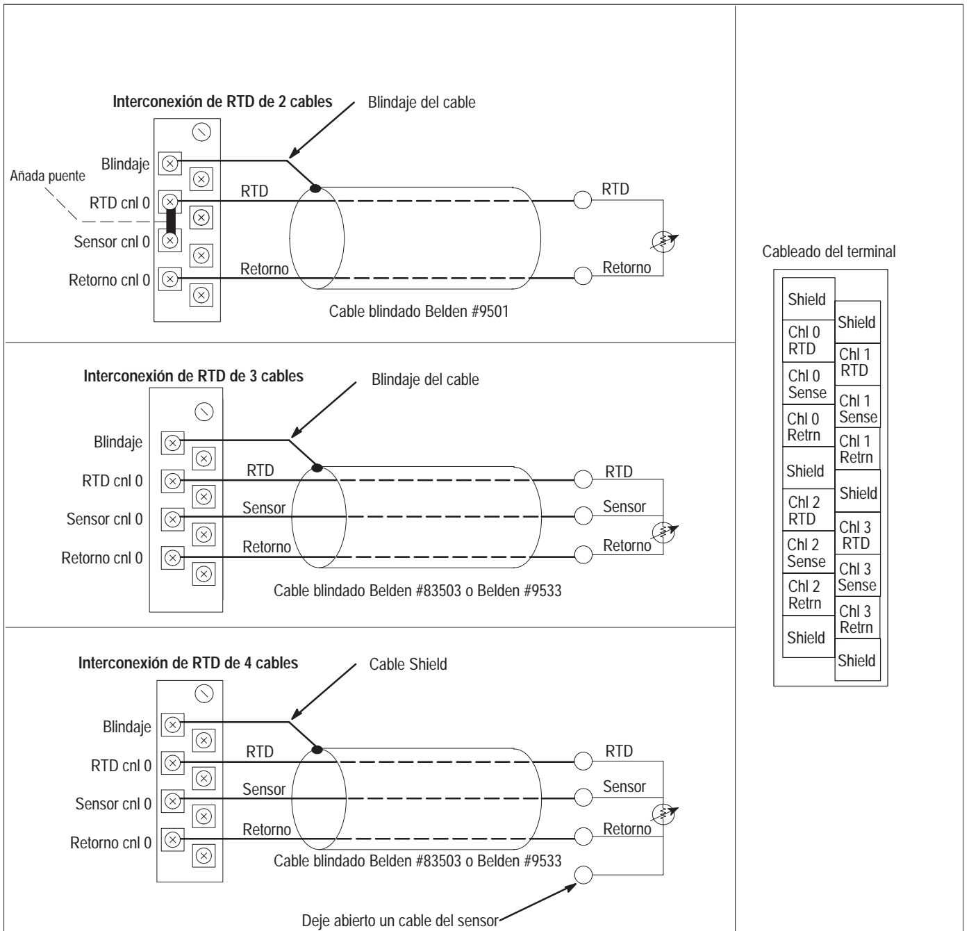
Figura 3.4 Conexiones de RTD al bloque de terminales
