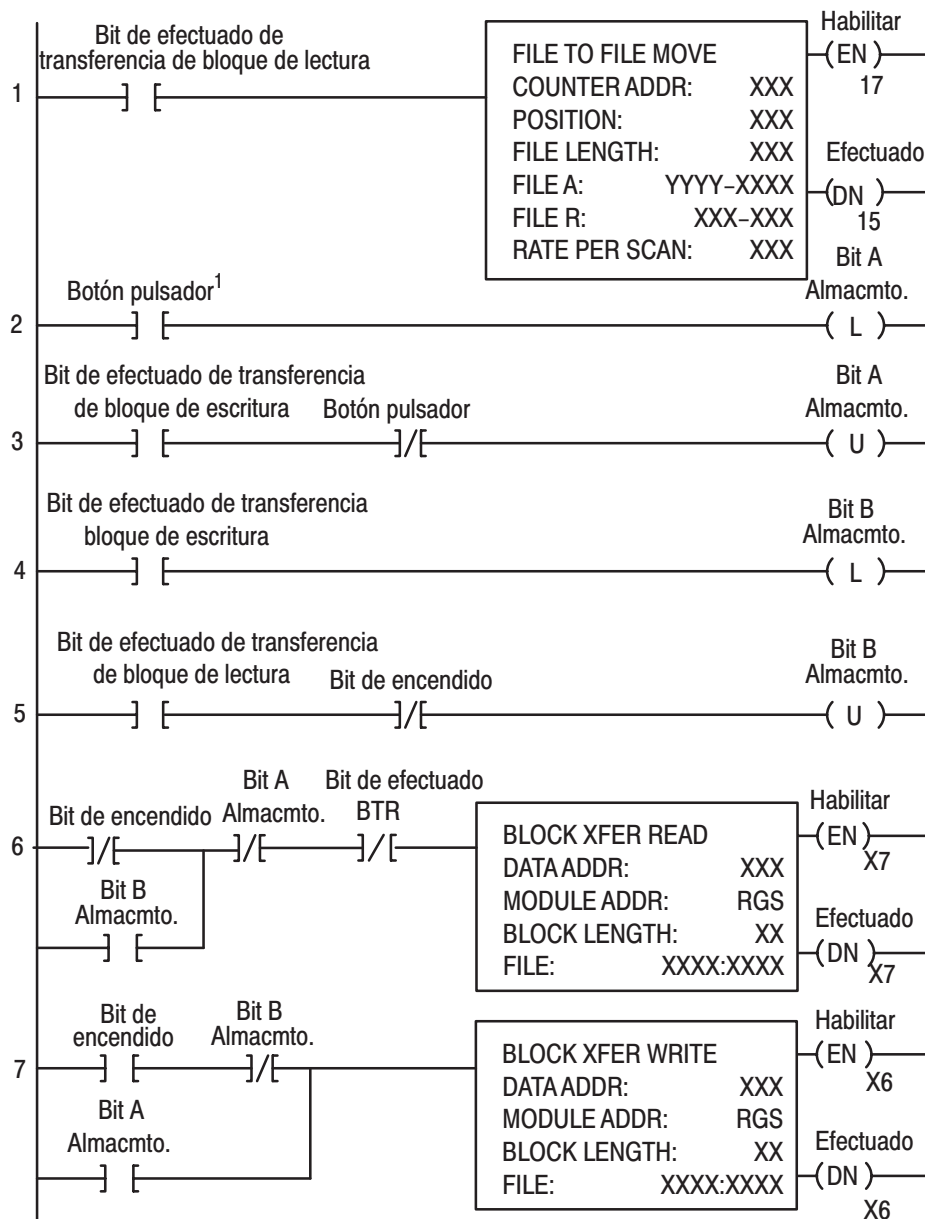
Figura 4.1 Estructura del programa de muestra de la familia PLC-2
