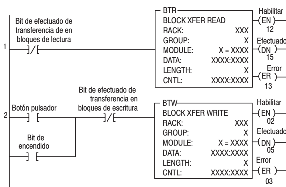
Figura 4.2 Estructura del programa de muestra de la familia PLC-3
